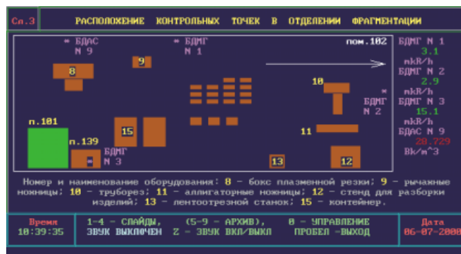
Рис. 2. Мнемосхема отделения фрагментации
